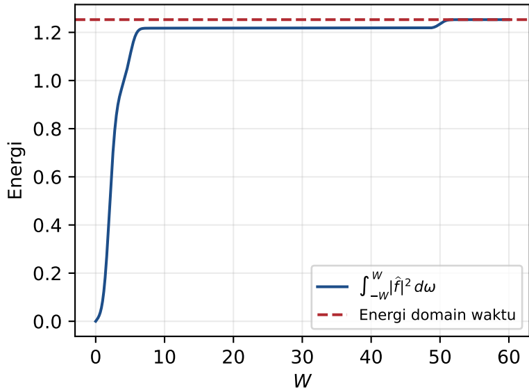
Pemeriksaan Plancherel
