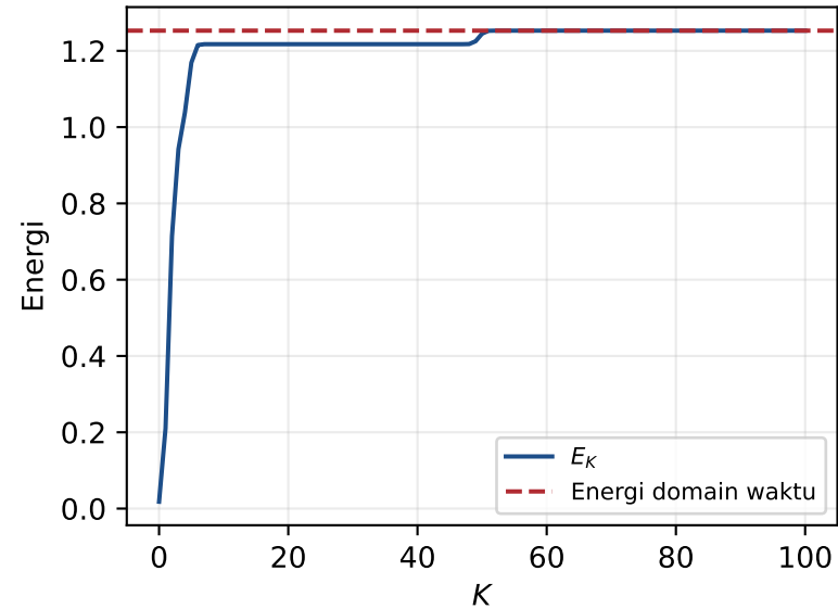
Pemeriksaan Parseval
